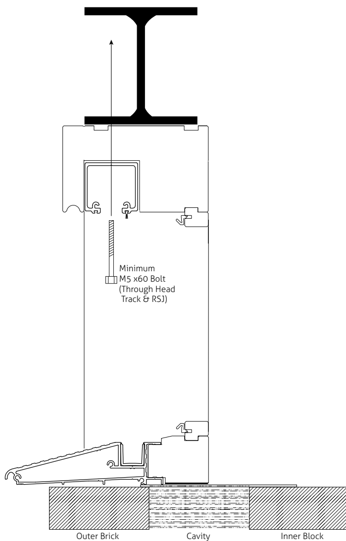
RSJ LINTEL
